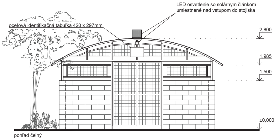
pohľad čelný
