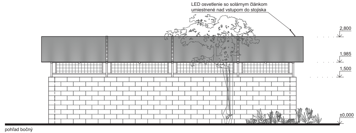
pohľad bočný
