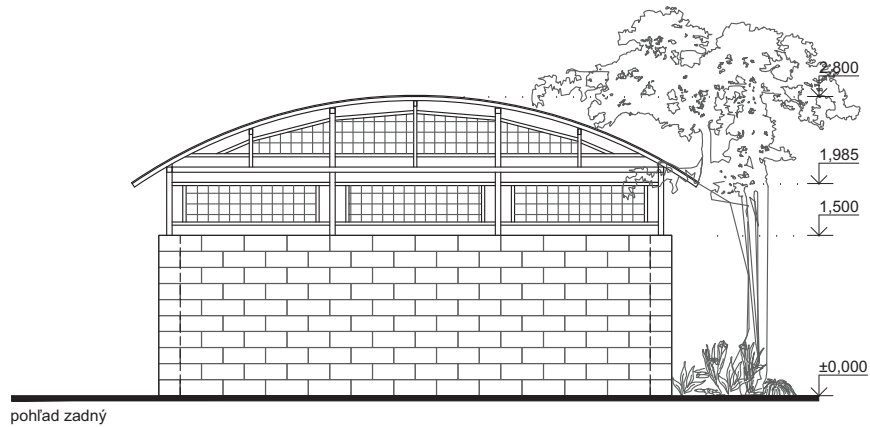
pohľad zadný
